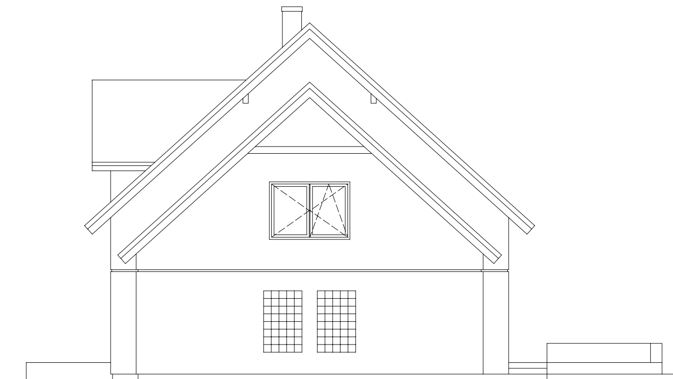
ELEWACJA PRAWA
