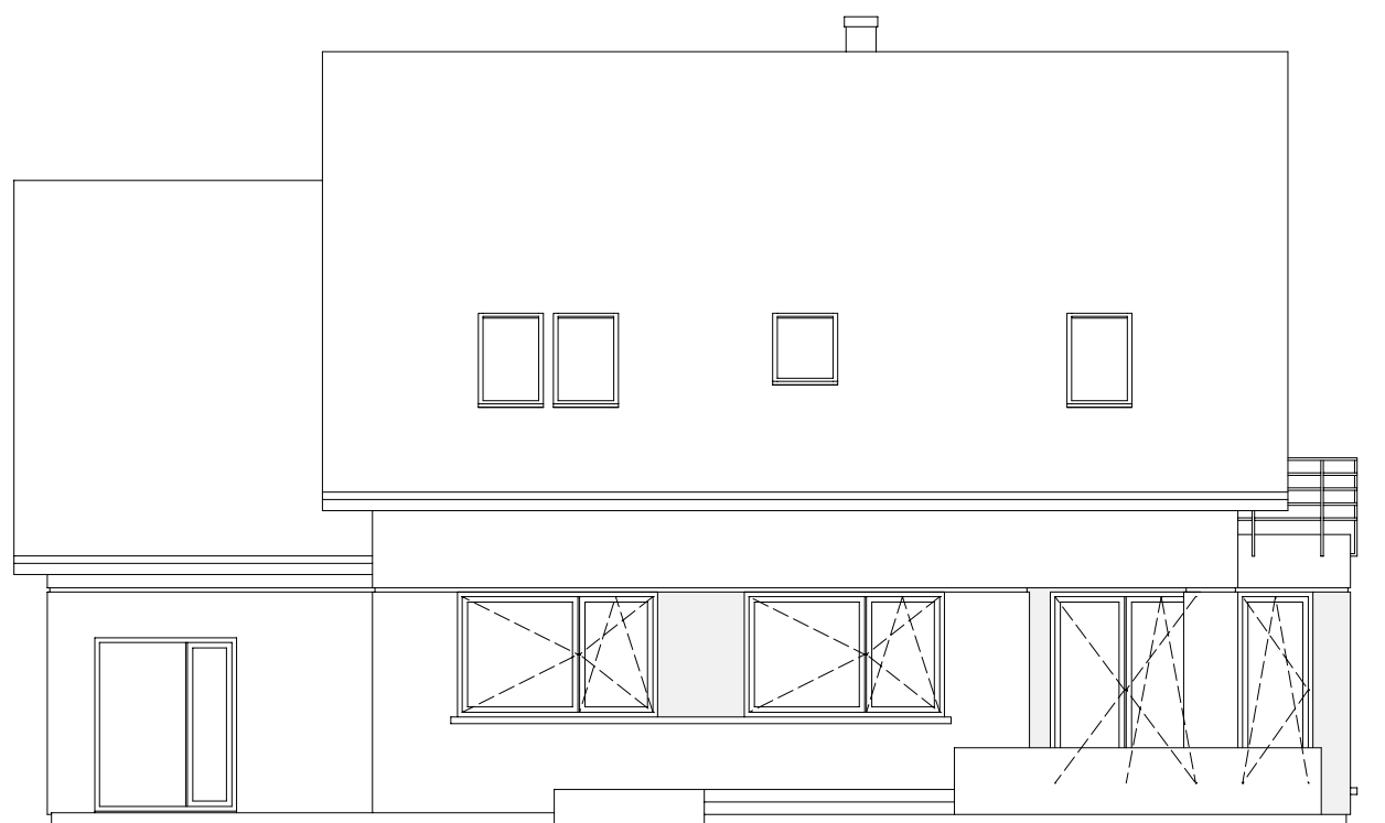
ELEWACJA OGRODOWA
